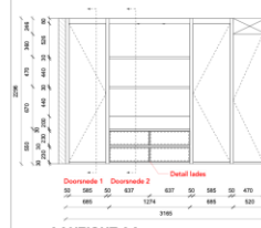
AANZICHT AA
