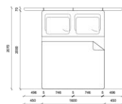
BOVENAANZICHT BED
