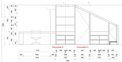
AANZICHT CC
