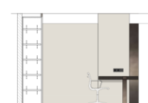
AANZICHT BB
