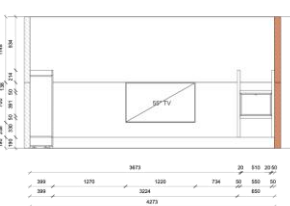
AANZICHT DD
