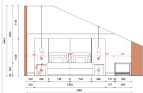
AANZICHT AA
